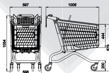
CPADF19508 19,5 kg.
