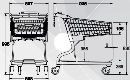
CPGSP09008 20,4 kg.
