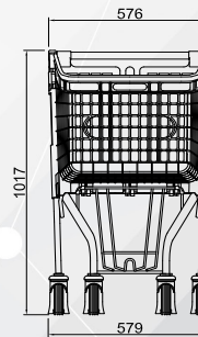
CPMASP1008 13,4 KG
