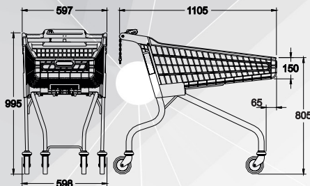
CPASP11008 16,4 kg.
