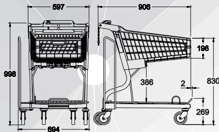
CPBSP09008 23,1 kg
