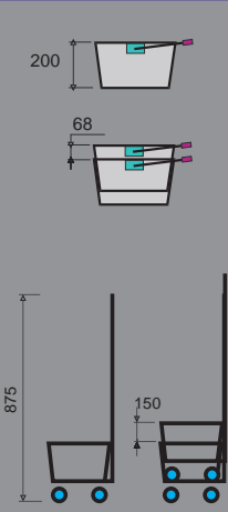
CHARIOT POUR RANGEMENT DE PANIERS BASKET STACKING TROLLEY
