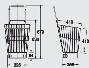
CHARIOT POUR RANGEMENT DE PANIERS BASKET STACKING TROLLEY
